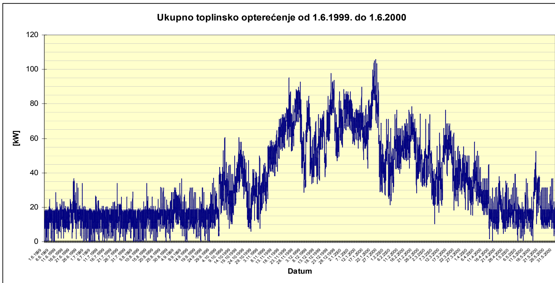
Slika 23. Dijagram ukupnog toplinskog opterećenja tijekom perioda od godine dana
