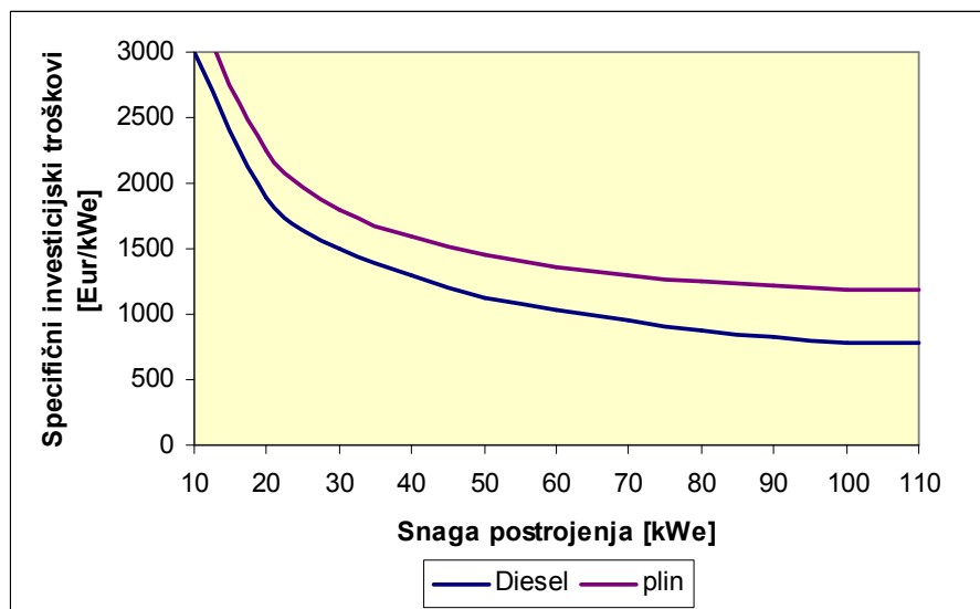
Slika 29. Ovisnost investicijskih troškova kogeneracijskog postrojenja o električnoj snazi
