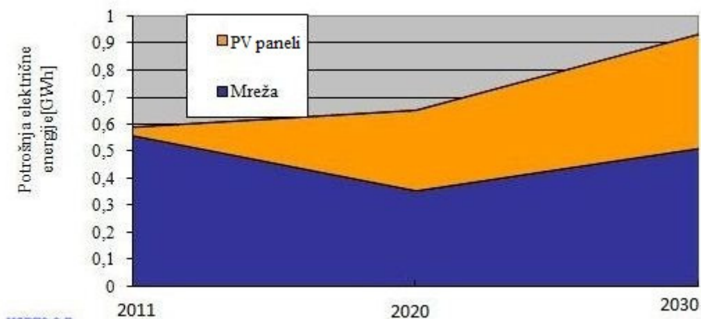
Dijagram 83. Dobava električne energije (PV otok)
